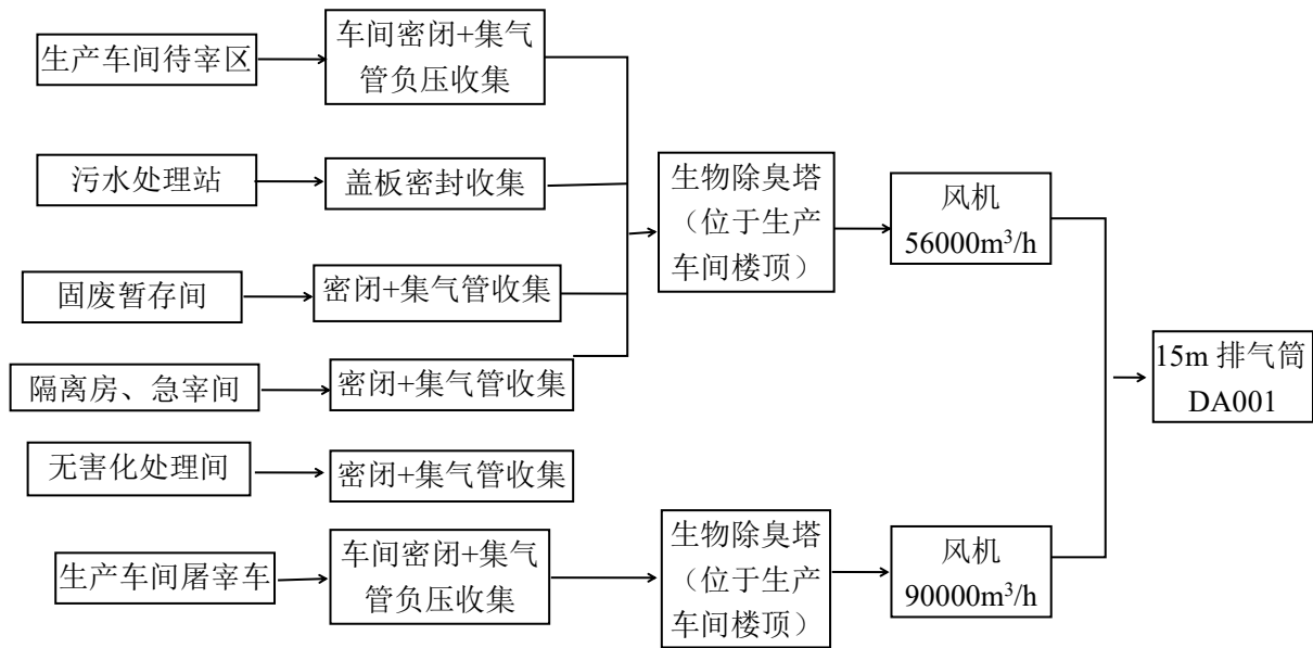
图 9.2.2-1 项目恶臭气体收集、处理流程图
