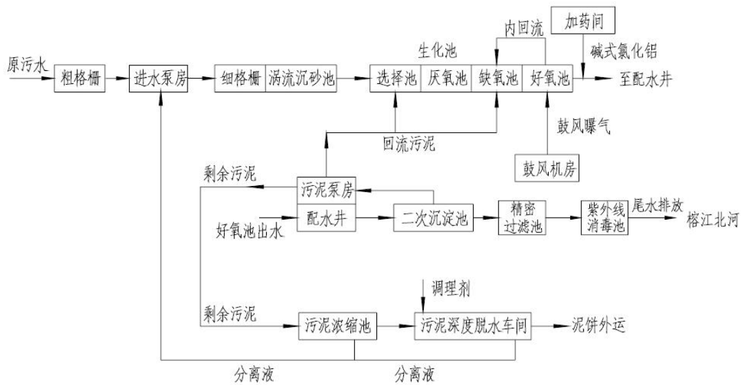
图 7.1-1 处理工艺流程图
