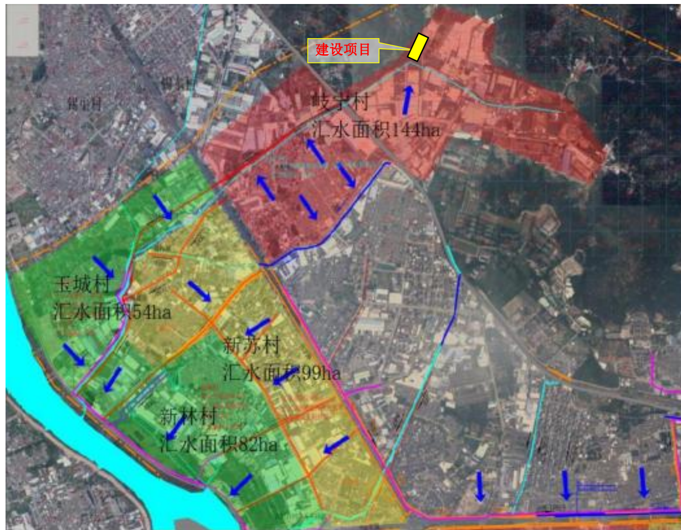
图 7.6.1-2 本项目所在片区截污管网及汇水方向示意图
