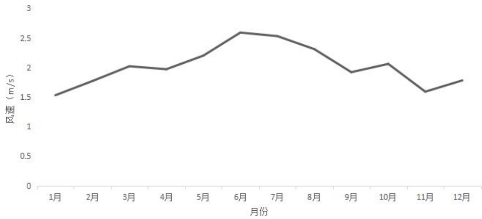
图 7.2.1-3 月平均风速变化曲线
