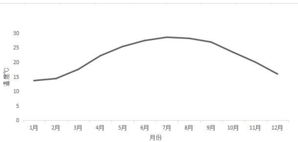
图 7.2.1-2 年平均气温月变化曲线
